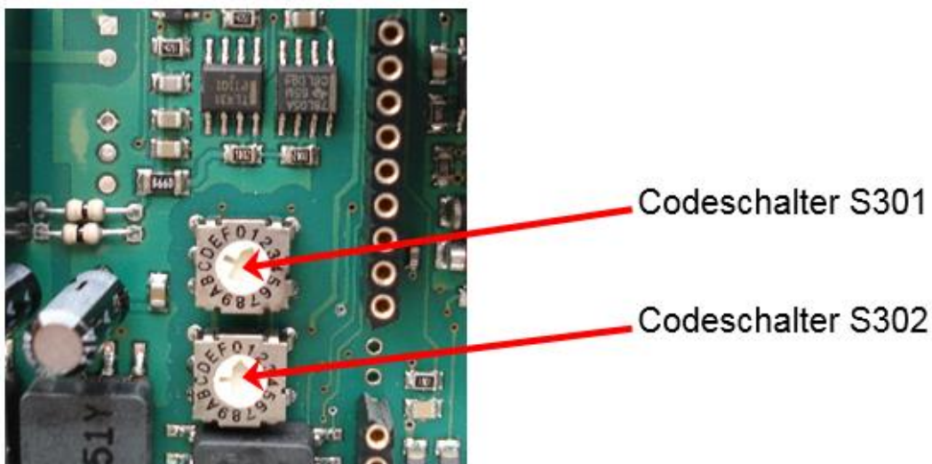
Abbildung 4 Drehschalter zur Einstellung von Adresse und Baud-Rate
