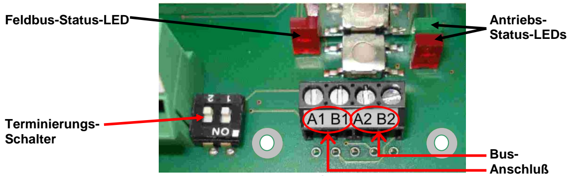
Abbildung 2 Klemmenblock auf der Hauptplatine des Antriebs für Feldbus-Anschluss
