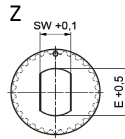
Zweiflach
