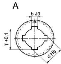
Passfedernut
