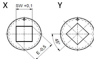
Vierkant
