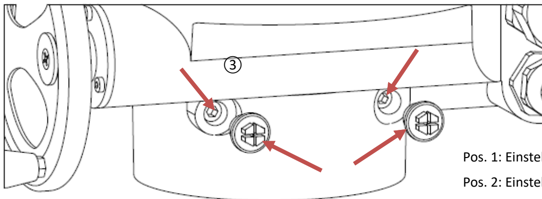
Abbildung 2: Mechanische Endlagenbegrenzung
