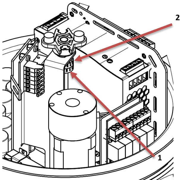
Abbildung 23: Einstellung Schaltnocken
