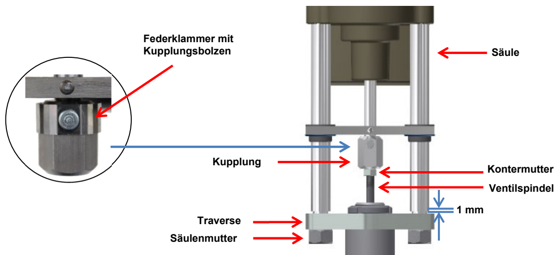
Abbildung 5: Armaturenanbau
