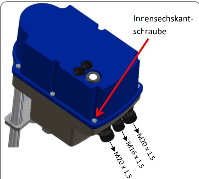
Abbildung 6: Öffnen und Schließen der Haube
