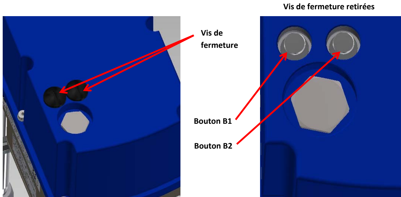
Figure 4: Commande manuelle pour les travaux de réglage dans les zones potentiellement d'explosives
