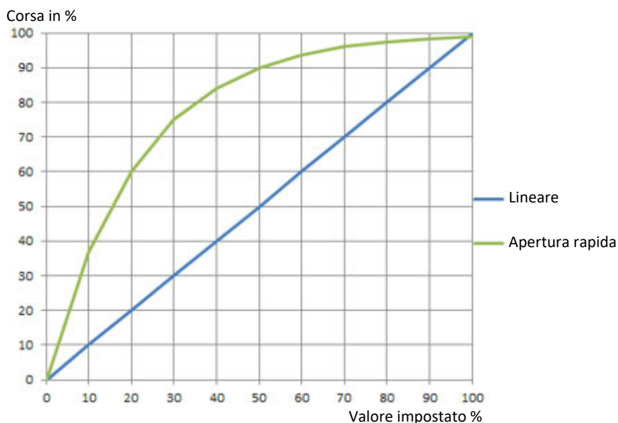
Figura 10: Curva della valvola
