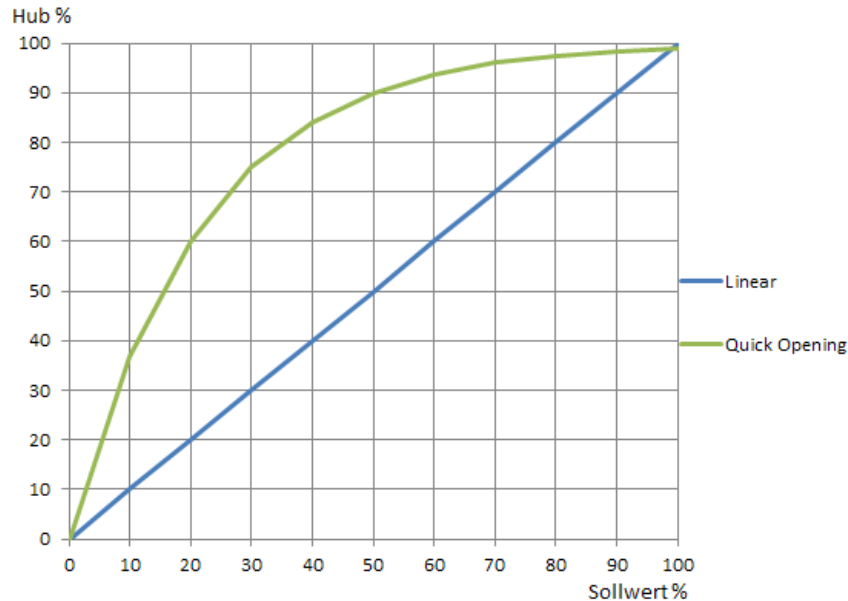
Abbildung 14: Armaturkurve
