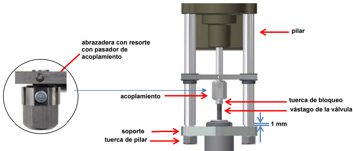
Figura 4: Montaje de la válvula
