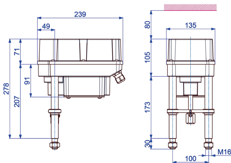
Abbildung 1: Einbaumaße
