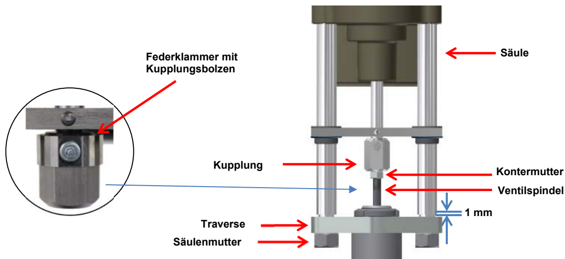
Abbildung 4: Armaturenanbau
