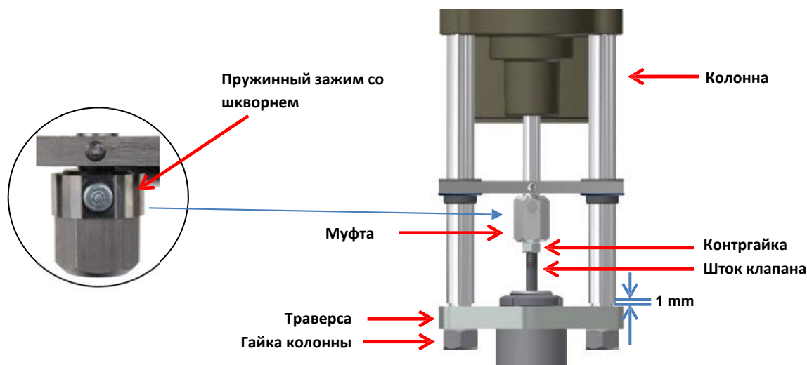
Рис. 4: Установка арматуры
