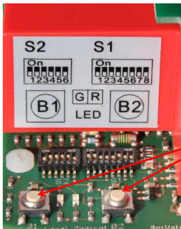
Рис. 3 Ручное управление
