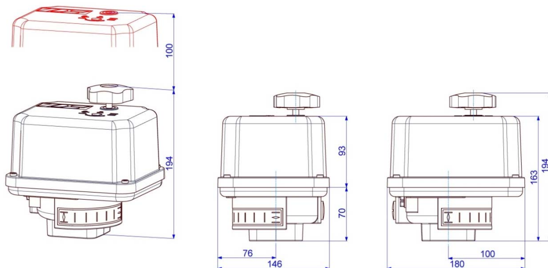
Рисунок 1: Установочные размеры
