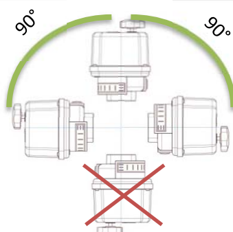
Рисунок 3: Положения установки
