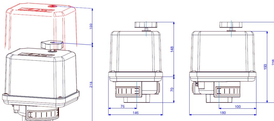
Рисунок 2: Вариант PSR-E 24 VDC 6 сек
